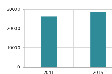
Nettoeinkünfte je veranl. Person 2011 und 2015
